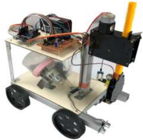
Fig.1. Hardware kit.
